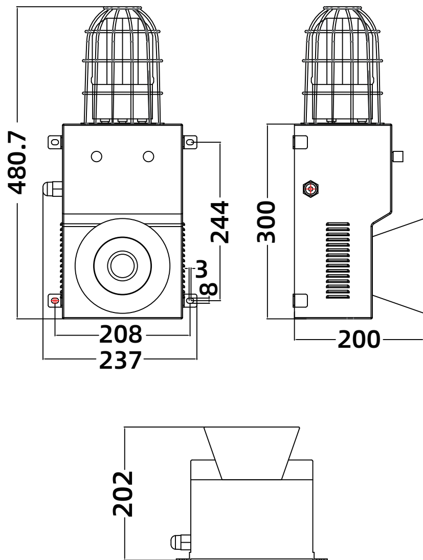
图2: HXA-SG2109尺寸图
